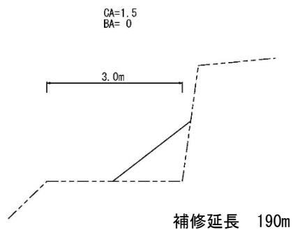
作業道補修標準断面図
