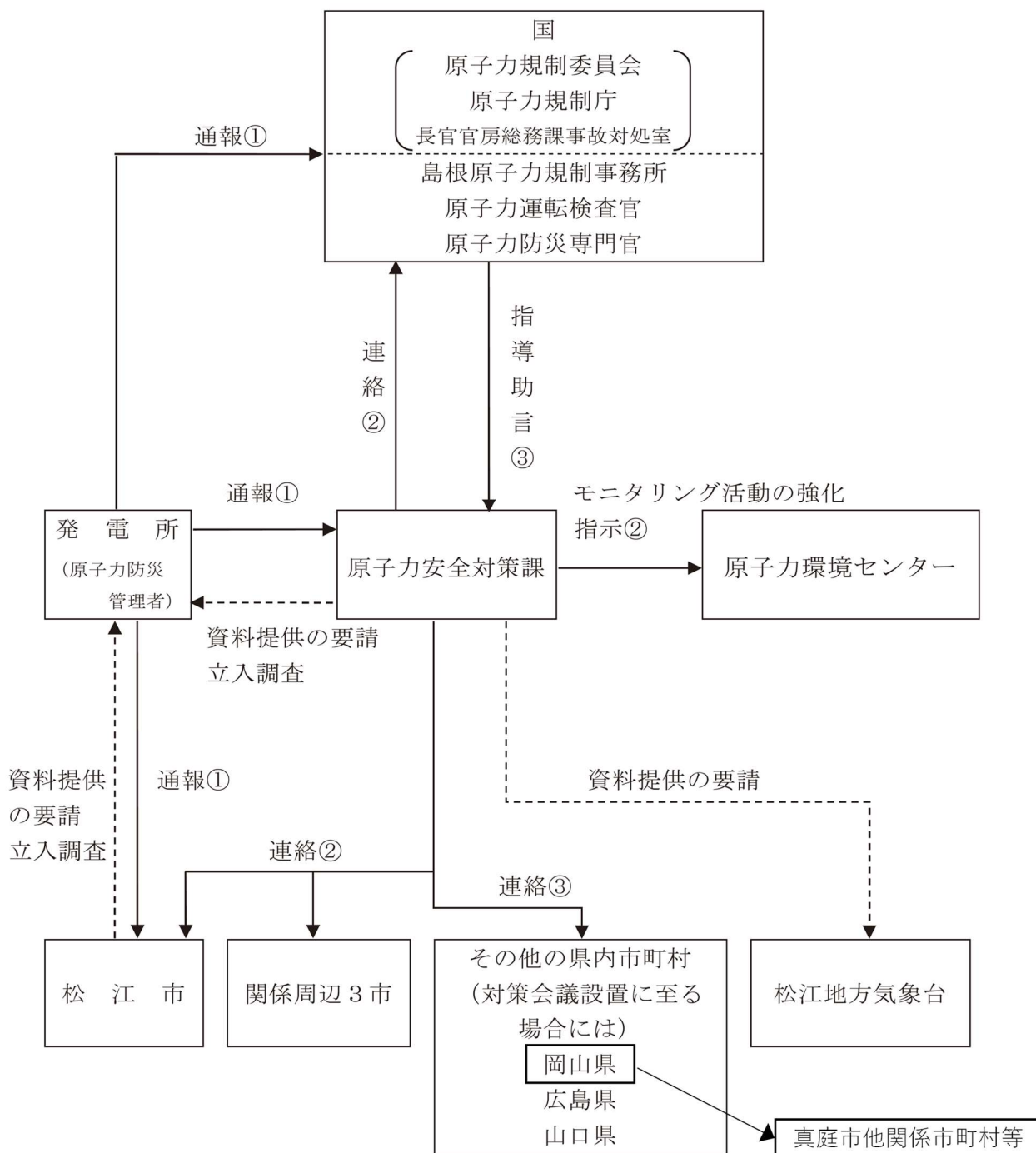
[島根県における発電所異常時連絡系統図]
