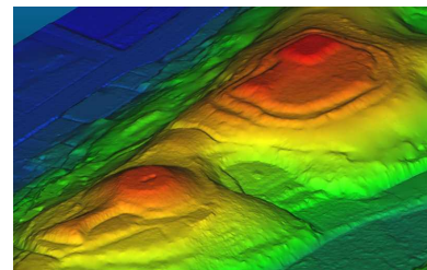
ドローンによる三次元測量調査で作成した鳥瞰図
